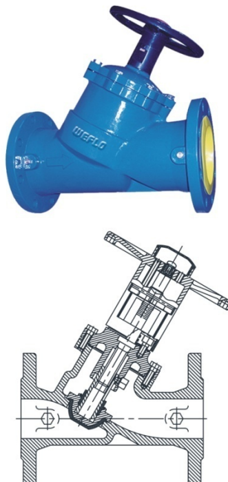
调节阀 2 及其剖析图
