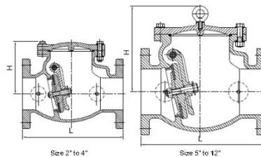
法兰旋启止回阀及其剖析图
