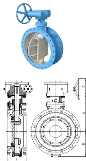
双偏心蝶阀及其剖析图
