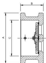
对夹双门止回阀及其剖析图
