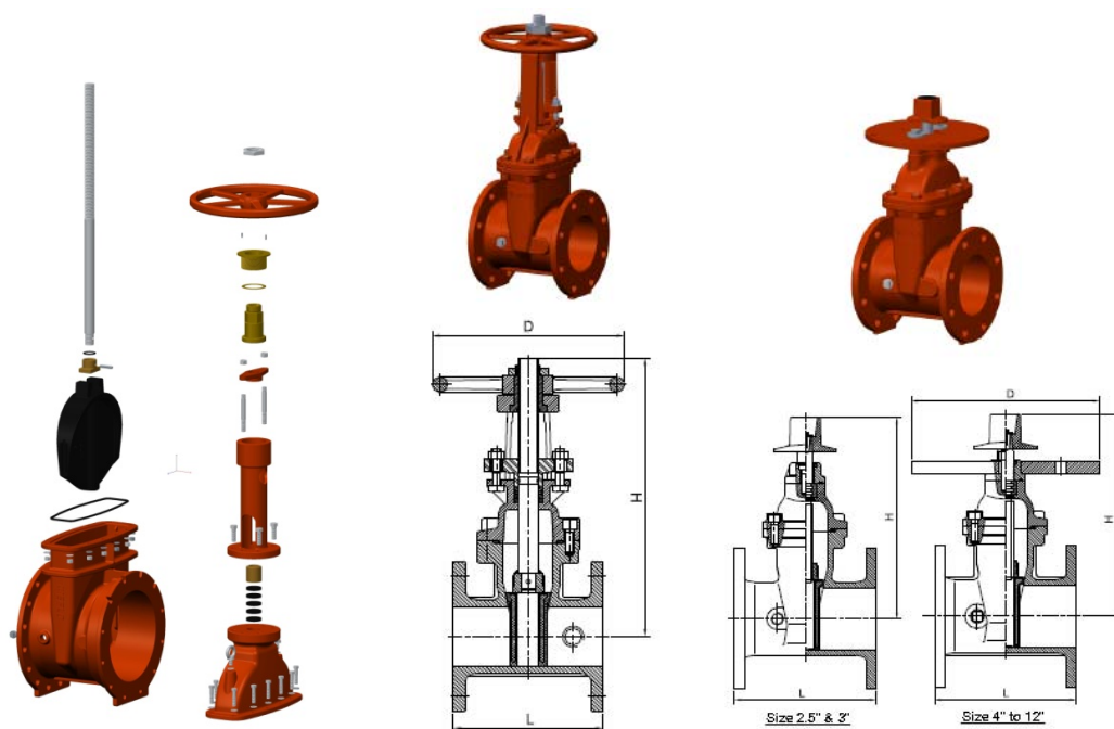
消防类明杆闸阀及其剖析图
