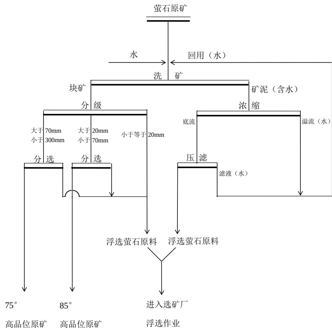
机器自动分选高品位萤石块矿预选的工艺流程如下图所示：
