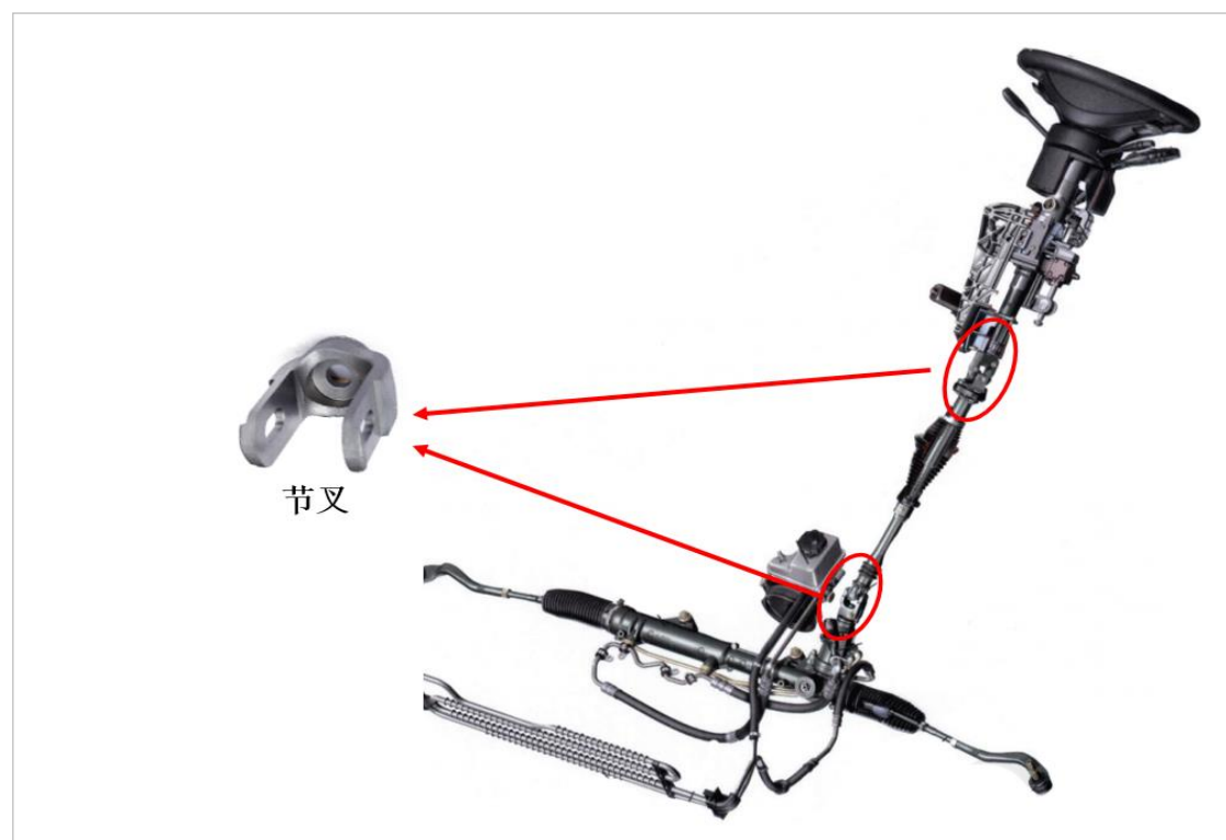
图：节叉在汽车转向系统中的位置示意图
