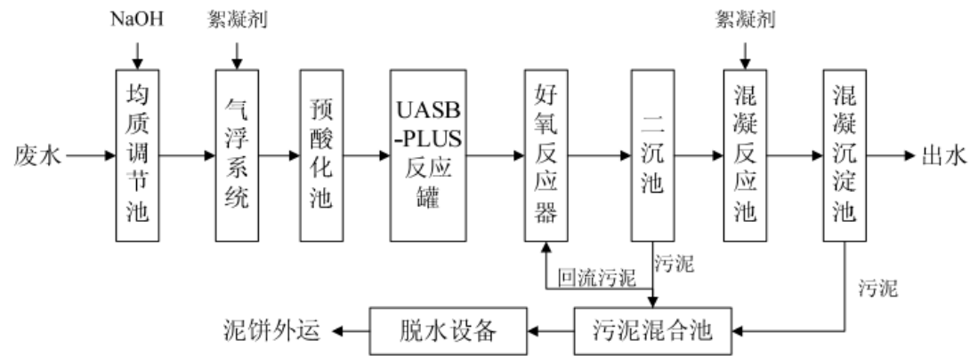
绿康生化污水处理工艺流程
