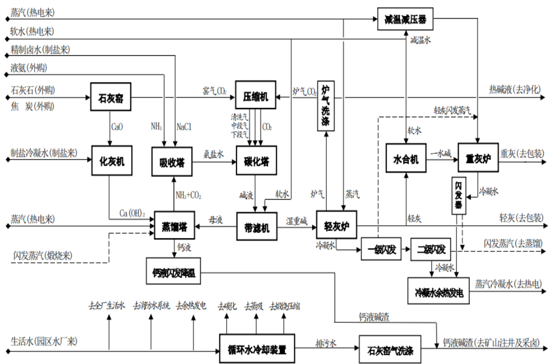
图 6.12 发行人纯碱生产工艺流程图
