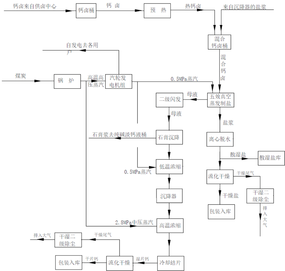
图 6.11 发行人盐钙联产工艺流程图
