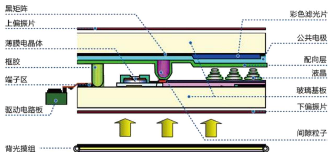
TFT-LCD 结构图
