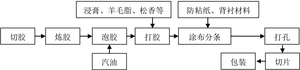
3、医用胶布胶带、绷带、运动保护产品生产流程图
