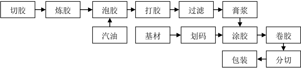
3、医用胶布胶带、绷带、运动保护产品生产流程图
