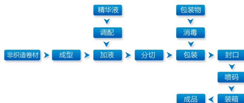
水刺非织造材料制品工艺流程
