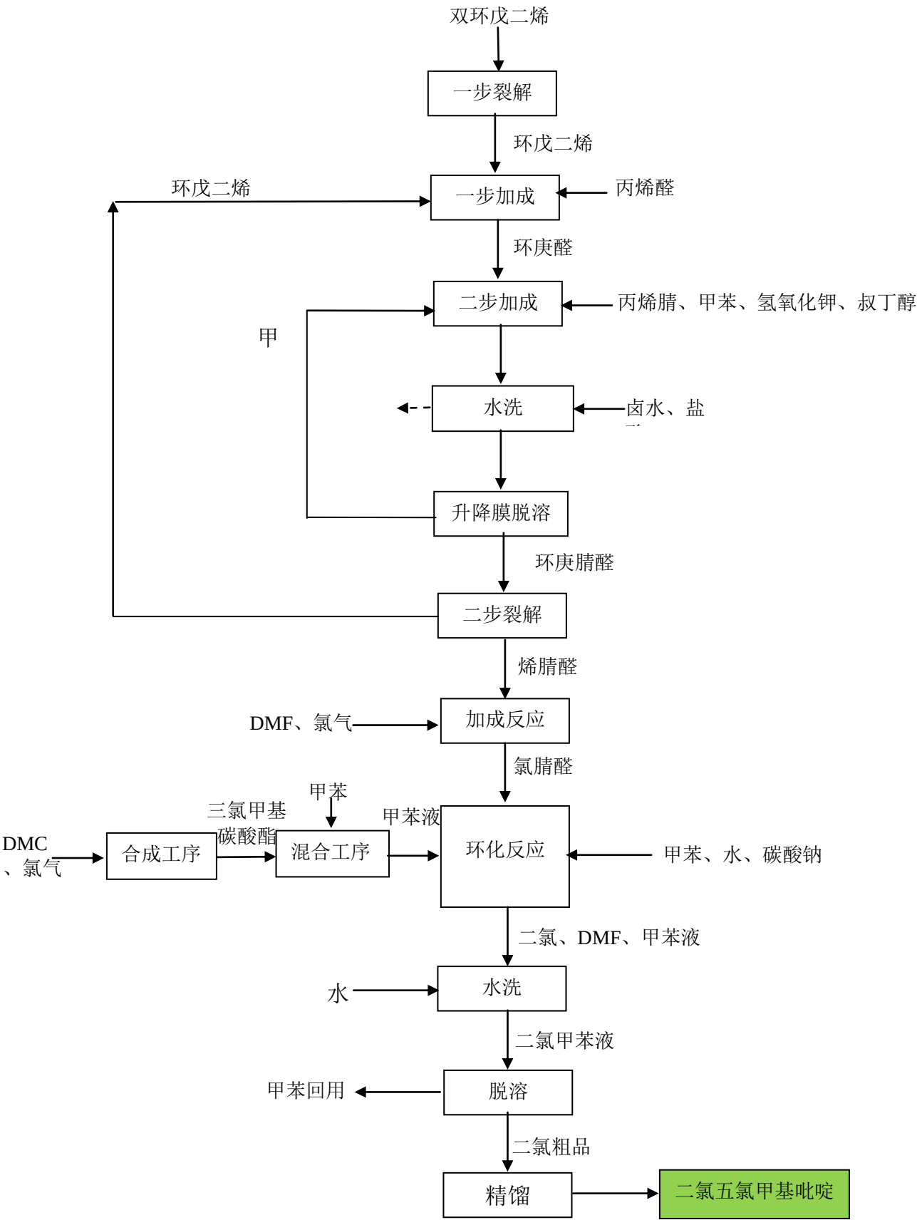
(2) 二氯五氯甲基吡啶生产流程图
