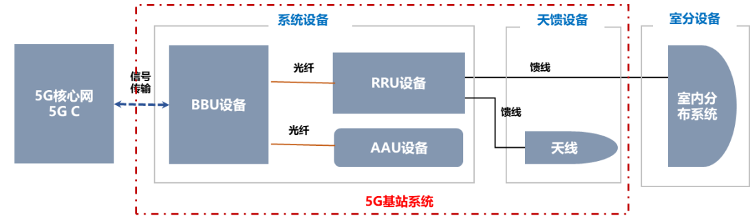
5G 移动通信网络设备简要示意图
