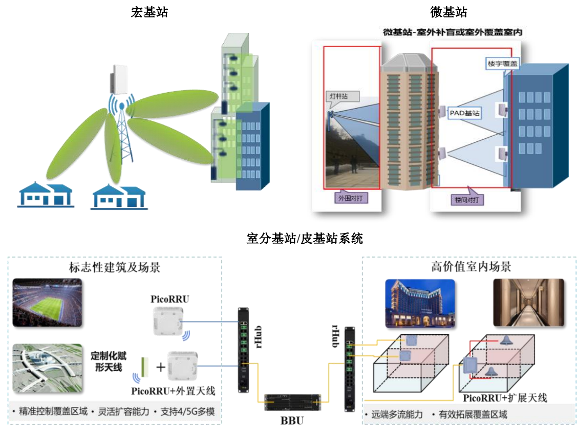
各类基站应用场景示意图
