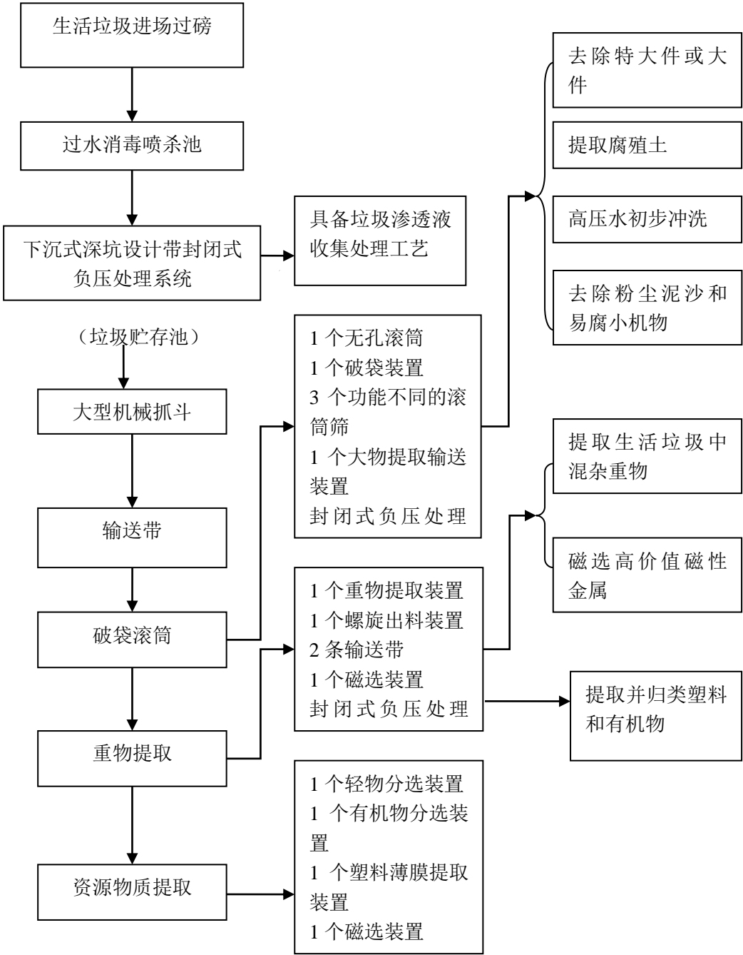
(2) 前端分选工艺流程图
