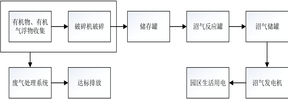
(7) 有机肥工艺流程
