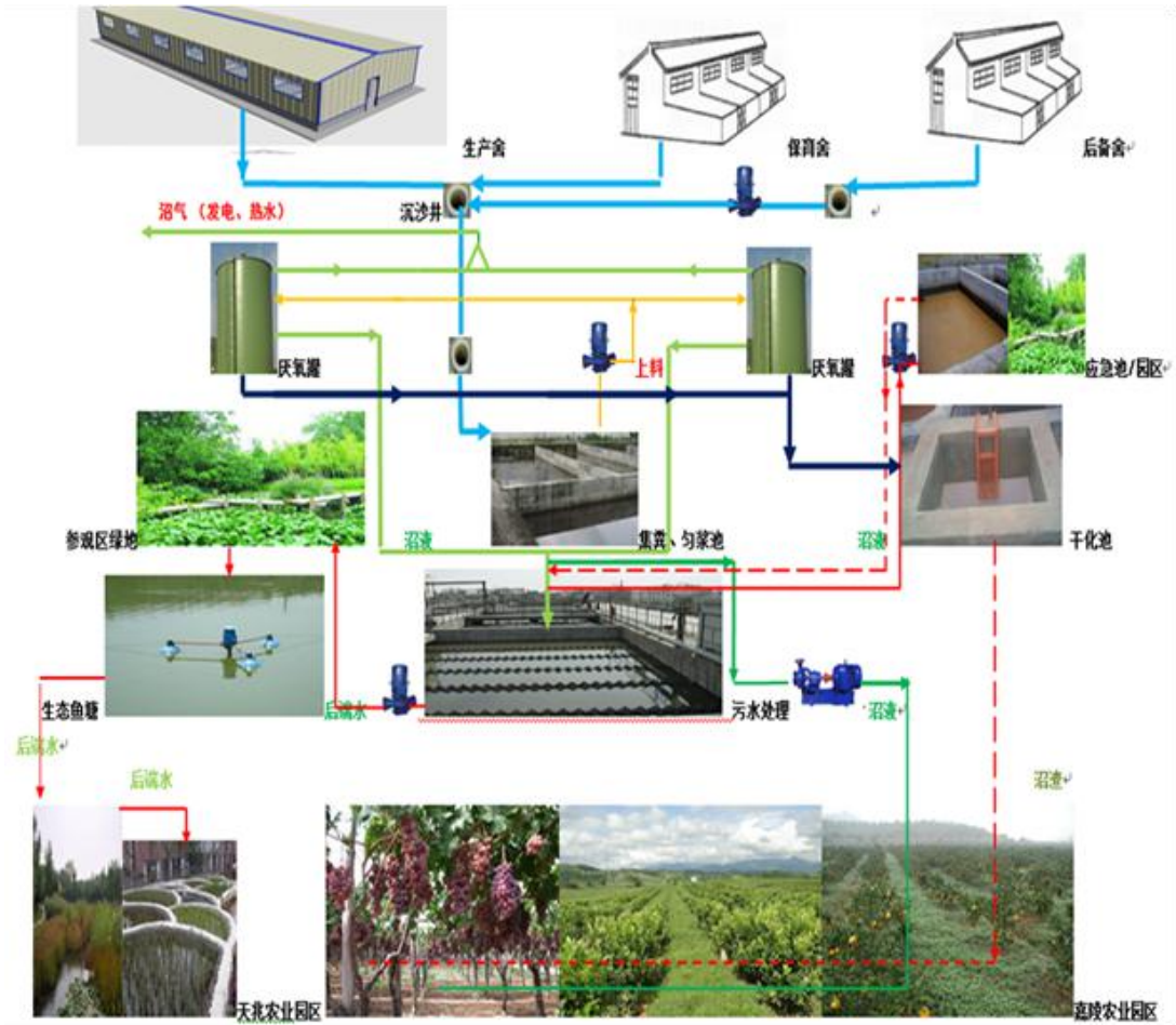
图：天兆猪业的污染物处理工艺流程图
