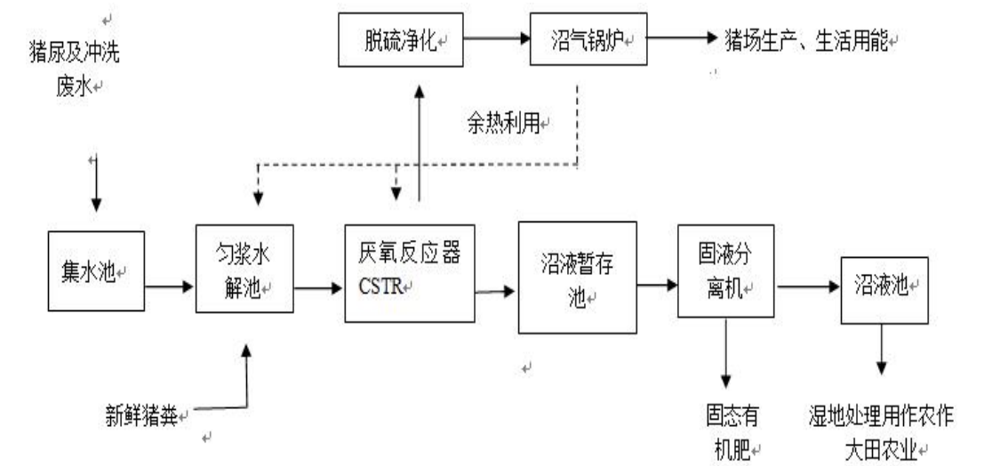
白坪猪场沼气工程工艺流程说明：
