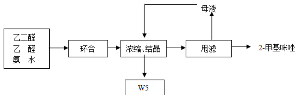
(4) 1, 2-甲基咪唑生产流程
