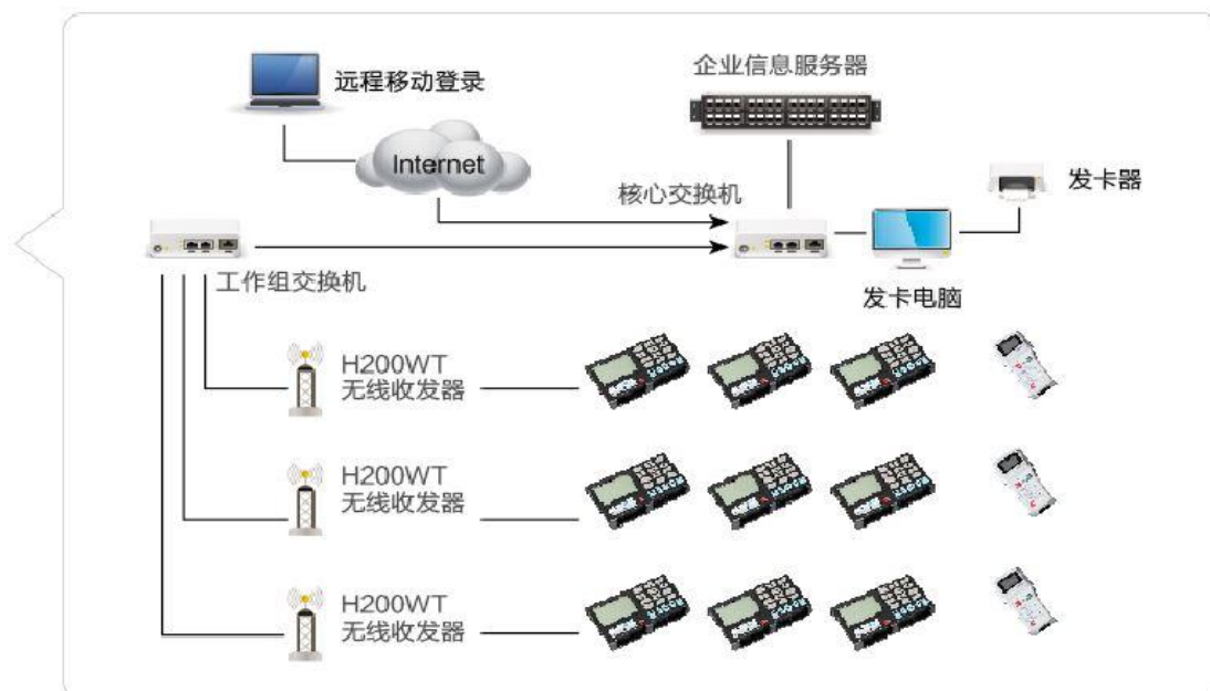
RFID 网络拓扑
