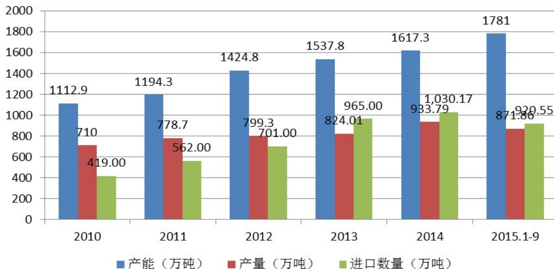
国内混合二甲苯产能、产量与进口情况
