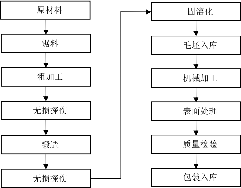
不锈钢管件产品生产流程图
