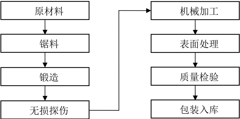
碳钢管件产品生产流程图
