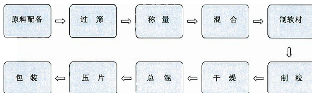
(3) 葵玛利健压片糖果生产工艺流程图
