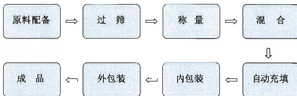
(3) 葵玛利健压片糖果生产工艺流程图
