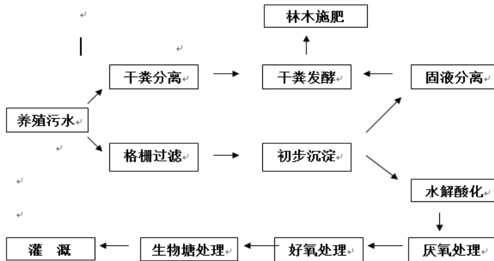
北川黑沟污水处理工艺流程图：
