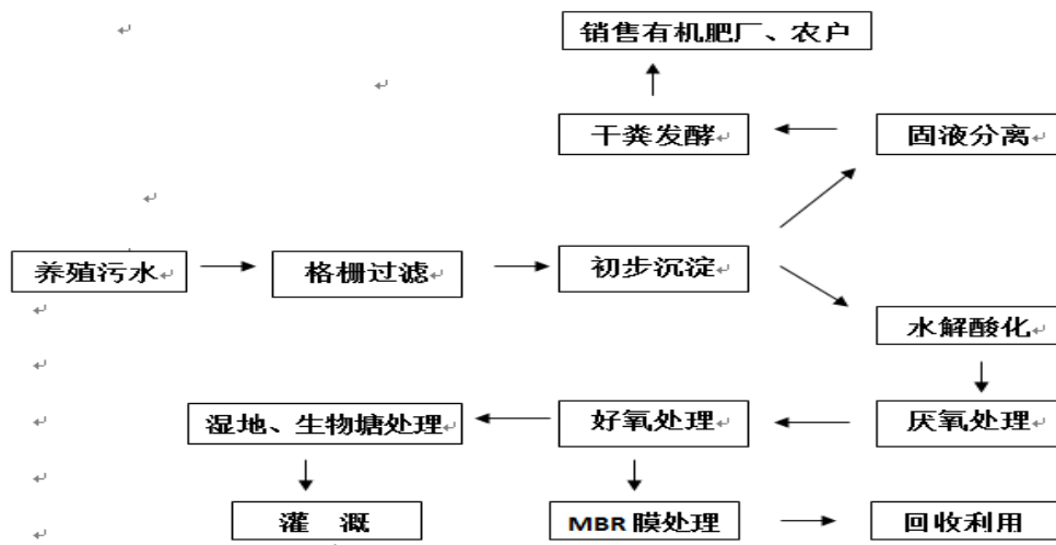
北川黑沟污水处理工艺流程图：
