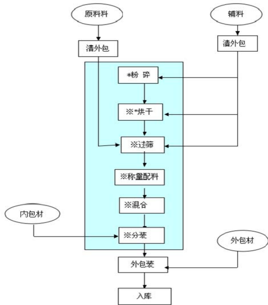
(4) 固体消毒剂工艺流程图
