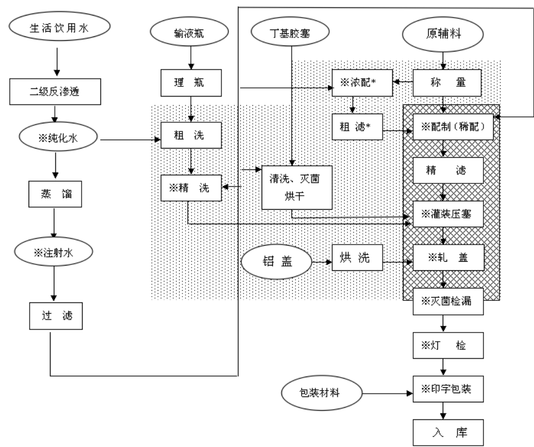
(2) 小容量注射剂工艺流程图
