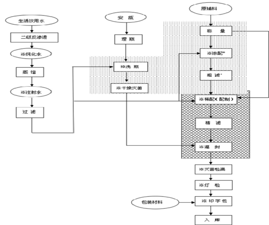
(3) 粉剂、预混剂工艺流程图
