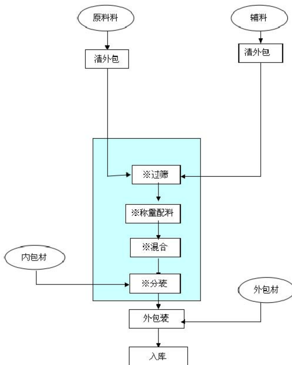
(5) 饲料添加剂、预混料工艺流程图
