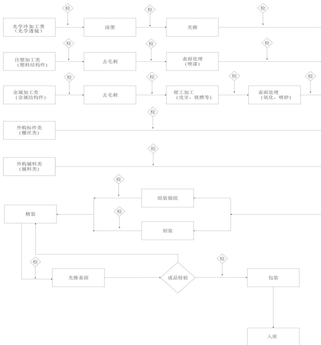
(2) 公司摄像机生产流程如下图所示：
