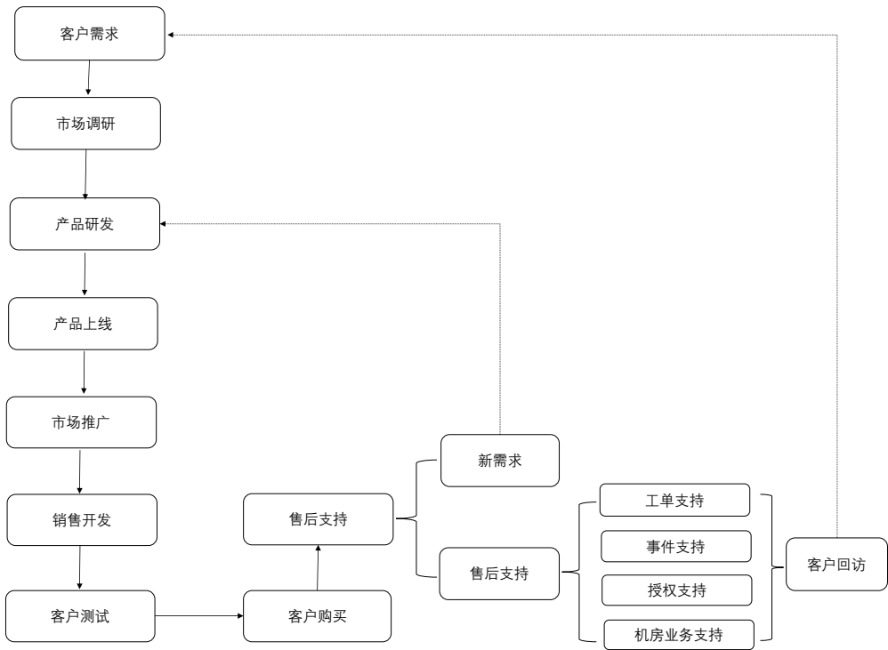
业务流程图
