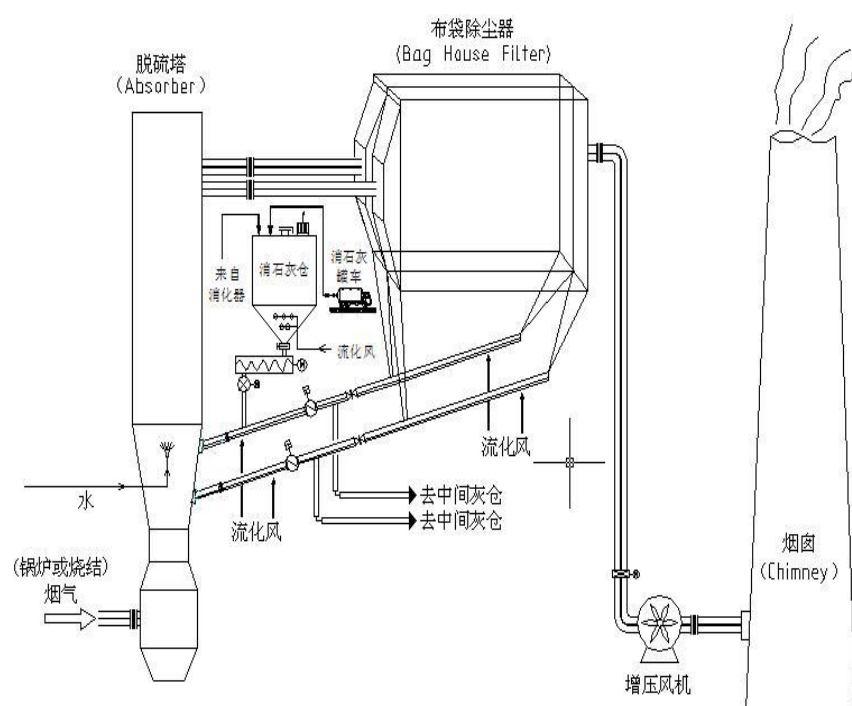
图三烟气处理流程
