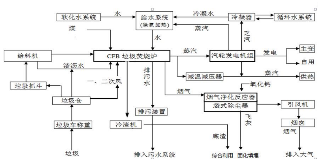
图二机械炉排式焚烧炉工艺流程
