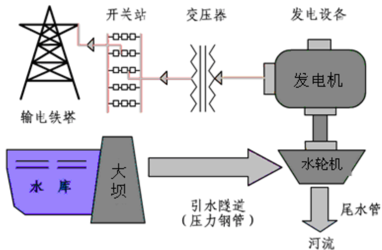
图 2-6 电力业务流程图
