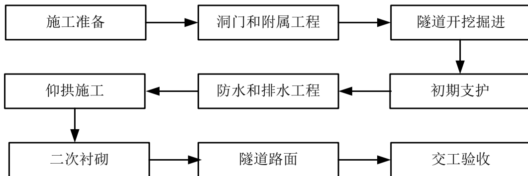
图 2-5 隧道工程施工流程图
