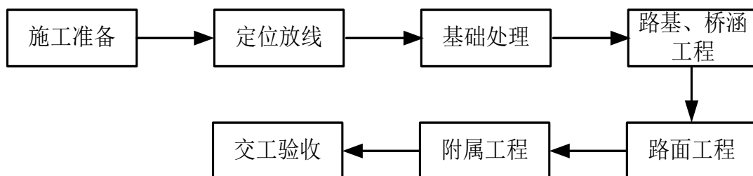
图 2-3 道路工程施工流程图
